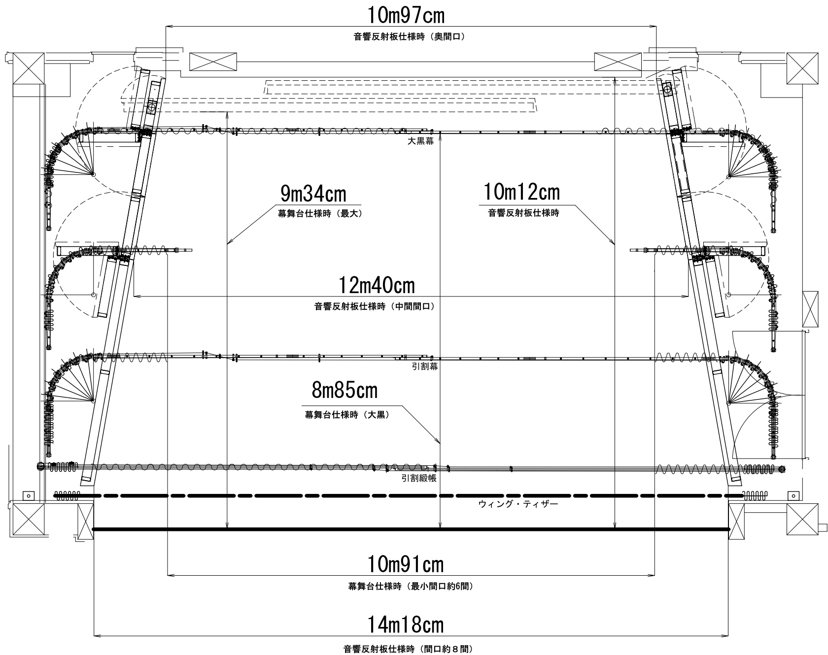
小田原三の丸ホール 小ホール 舞台形式（幕・音響反射板） 有効範囲
