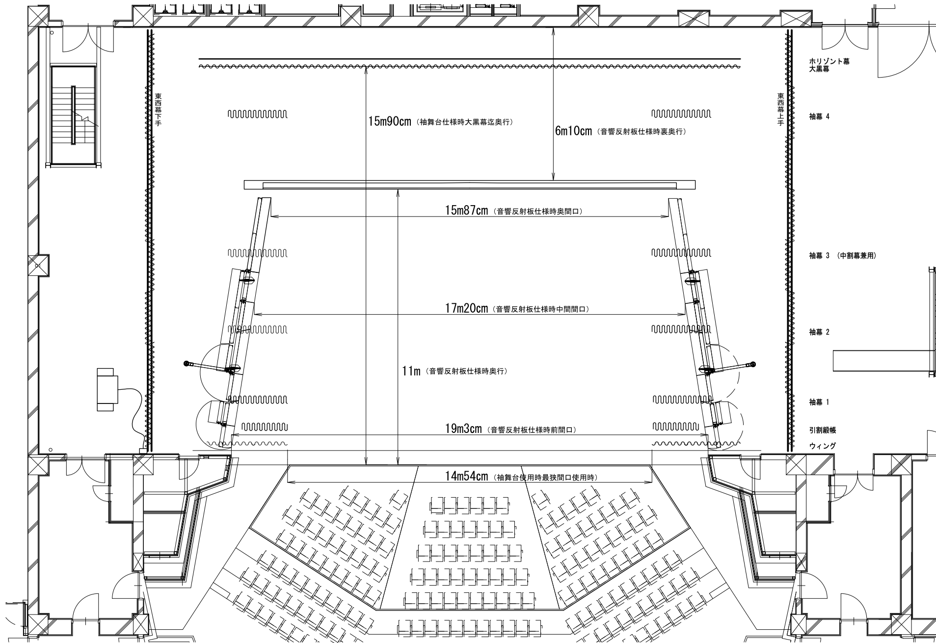
小田原三の丸ホール 大ホール 各仕様 有効範囲 平面図
