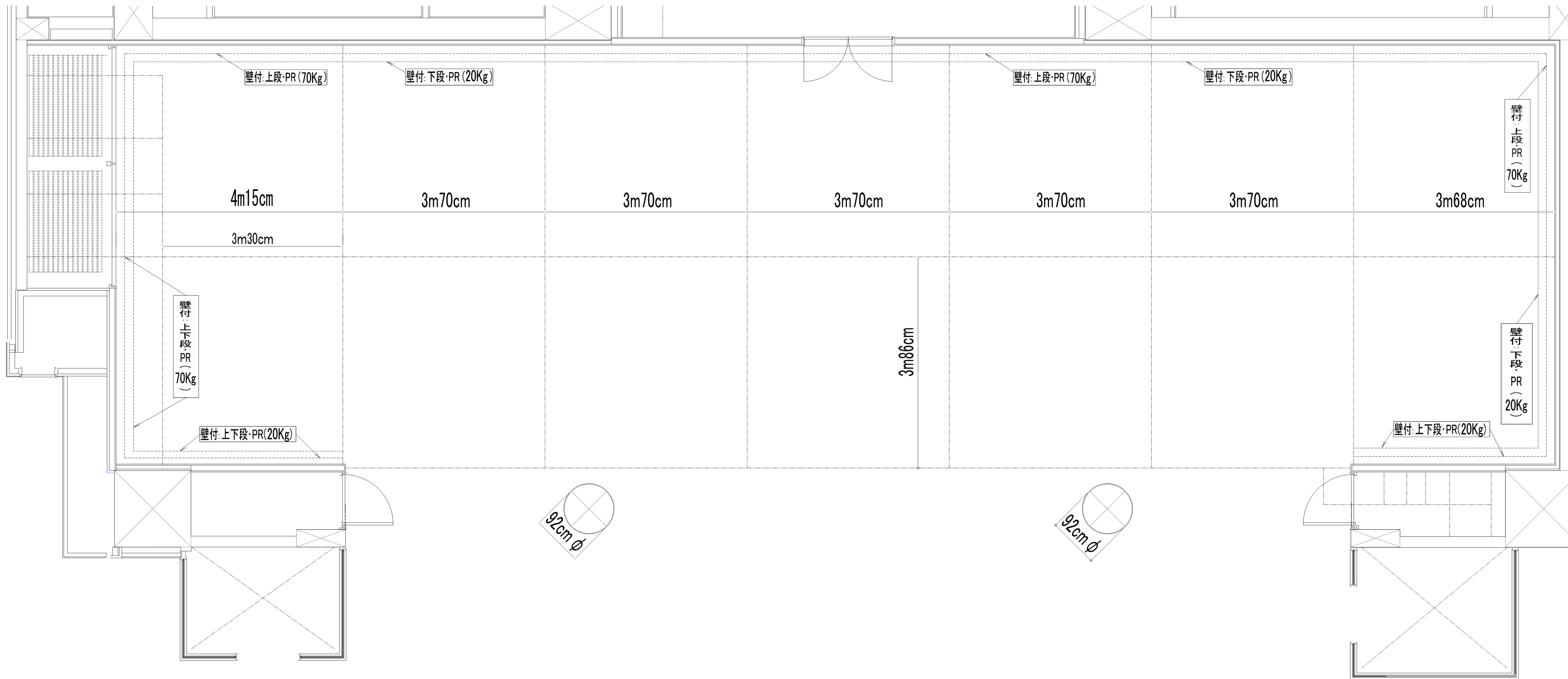
三の丸ホール 展示室 P.R耐荷重入り 平面図
