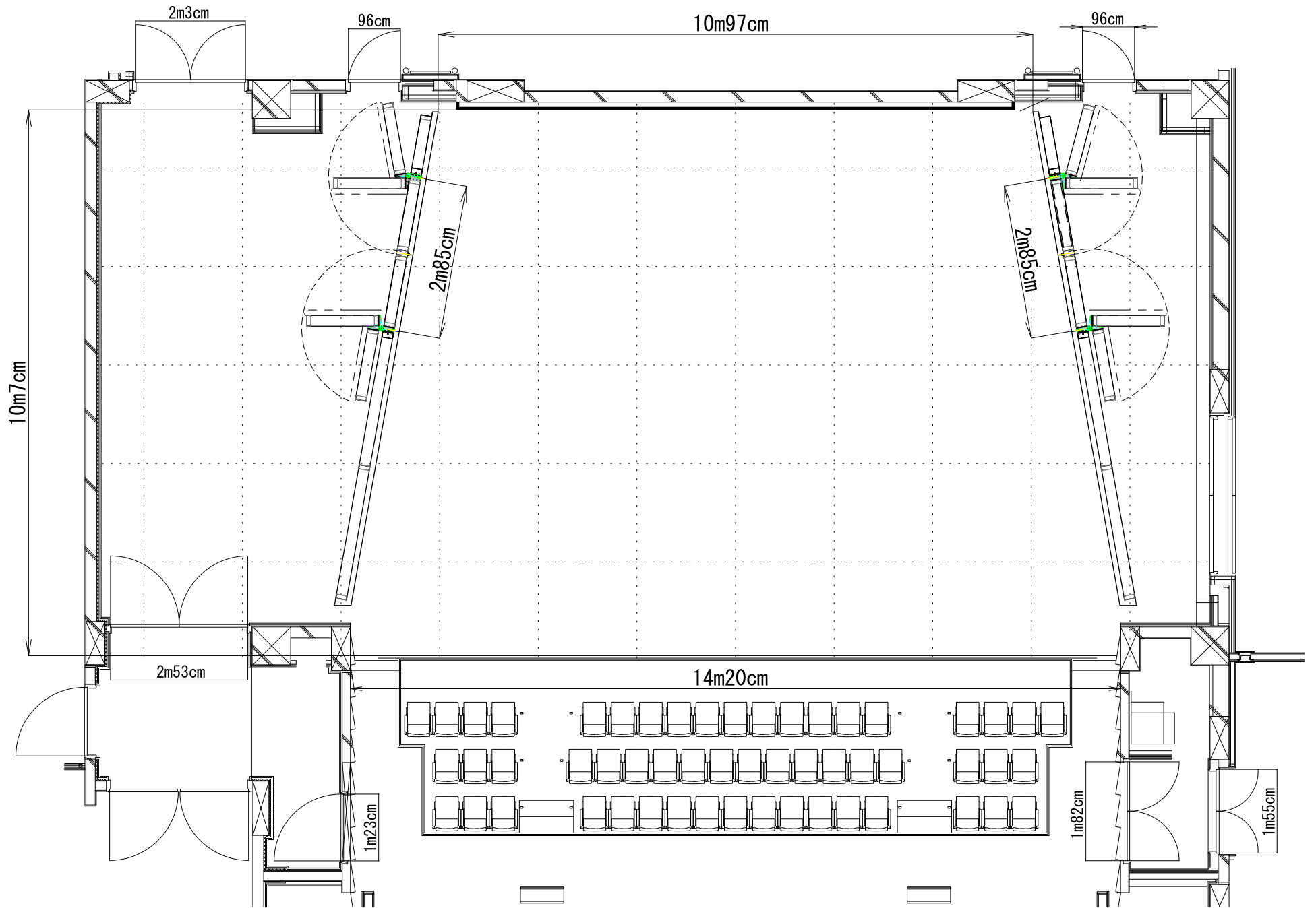
小田原三の丸ホール 小ホール 音響反射板平面図
